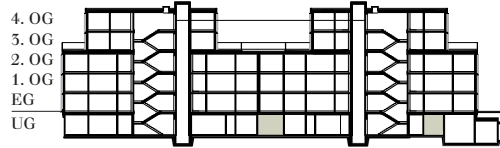
Schnitt
