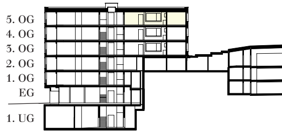
Schnitt
