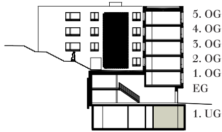
Schnitt
